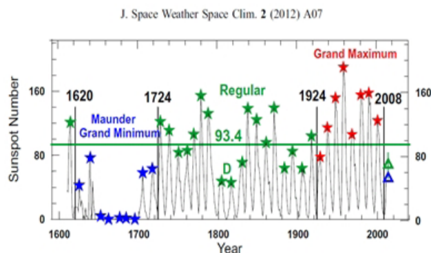
Gráfico de actividad y ciclos solares. / EPDA
