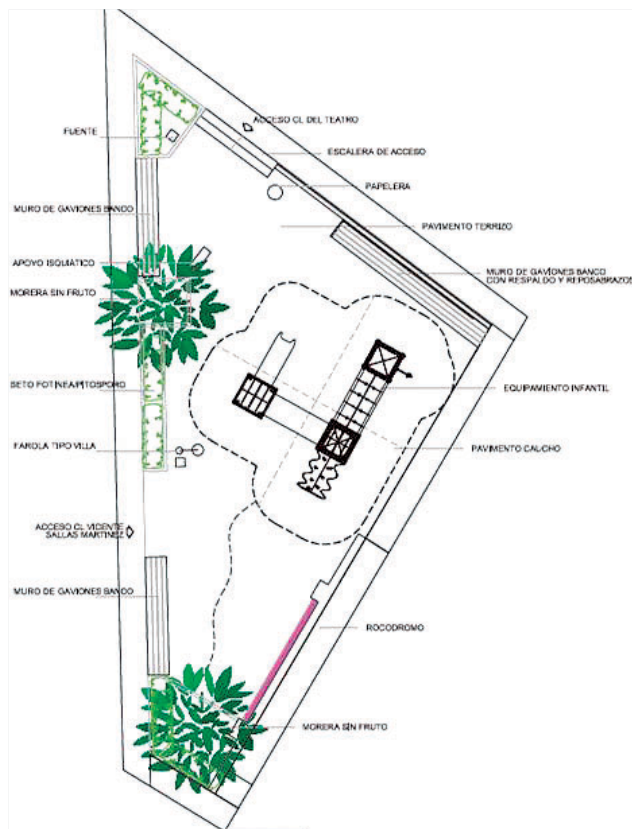
Alzado del proyecto para el parque. / EPDA
