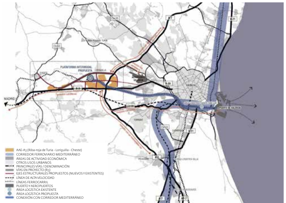
Planta general de ejes viarios y ferroviarios del entorno territorial del AAE A-3./ UPV
