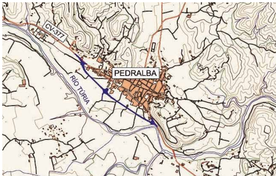
Situación del proyecto inicial de la variante sur de Pedralba en la CV-377. / EPDA
