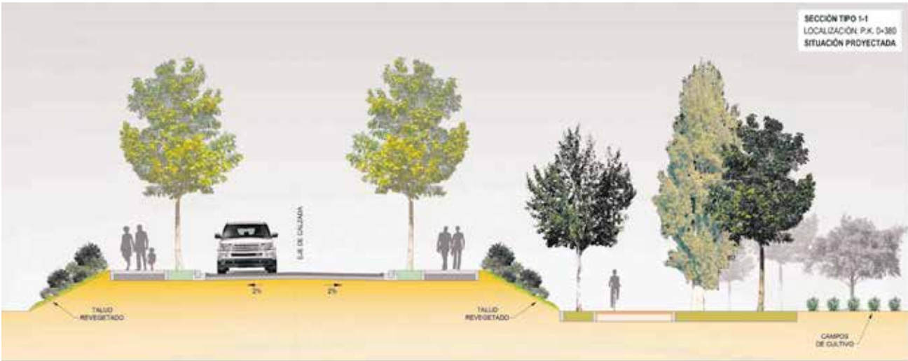
Plano de la sección transversal del corredor V-175 de Pedralba. / EPDA
