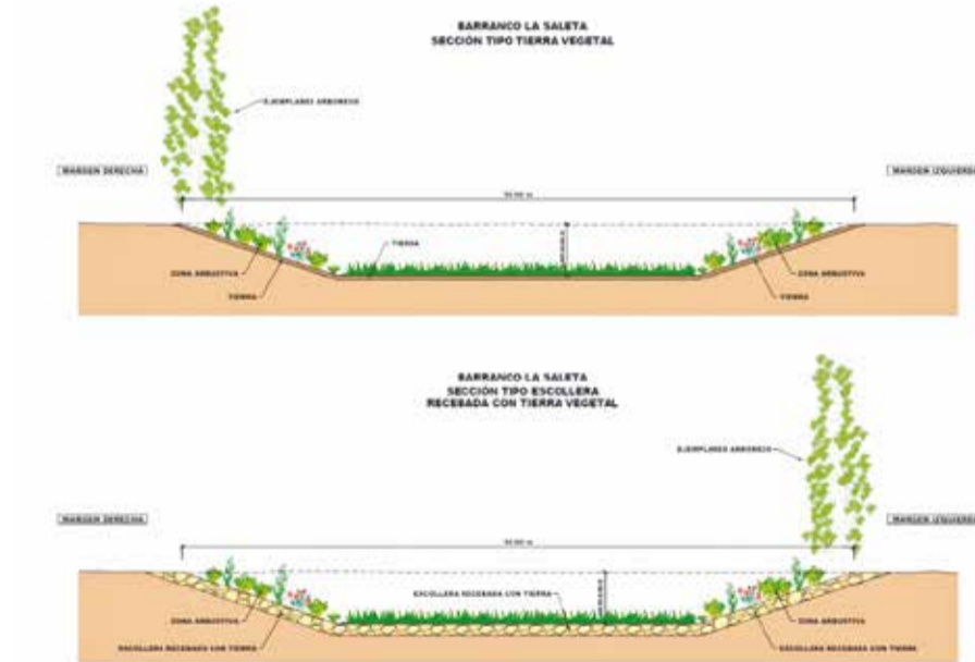
Figura 5. Via verde. Secciones tipo.
