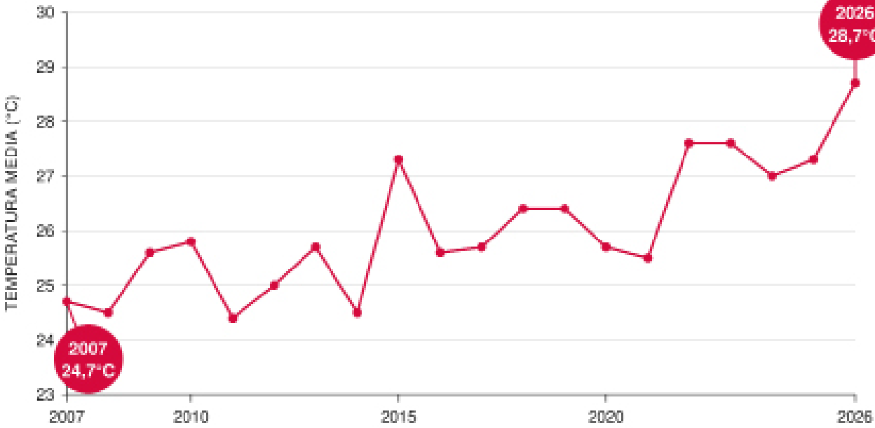
EVOLUCIÓN DE LA TEMPERATURA MEDIA DE JULIO EN LA ESTACIÓN DE CHESTE CENTRO
